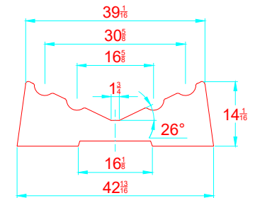
TRANSVERSAL SECTION "B" SECCION TRANSVERSAL "B"
