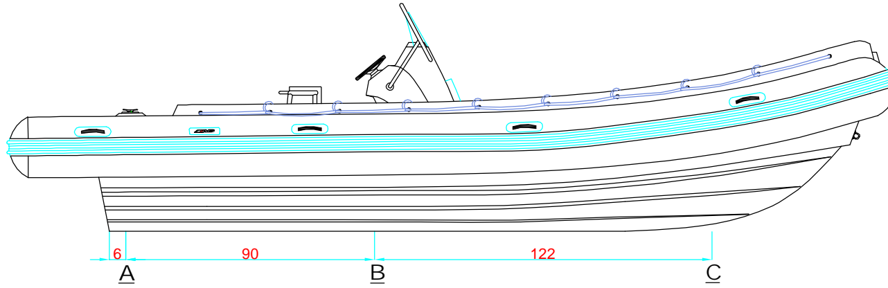
LONGITUDINAL PROFILE VISTA LATERAL
