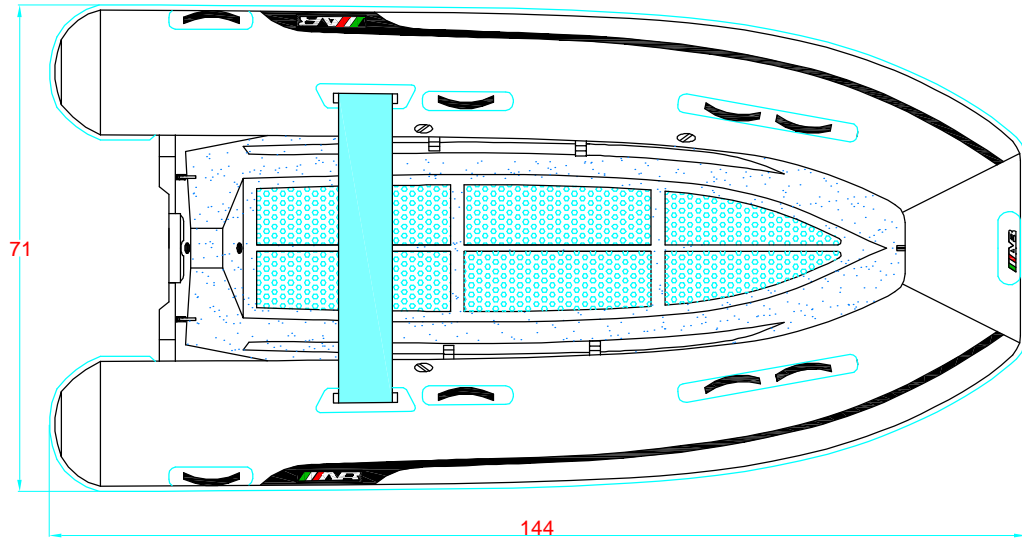
PLANT VIEW VISTA EN PLANTA
