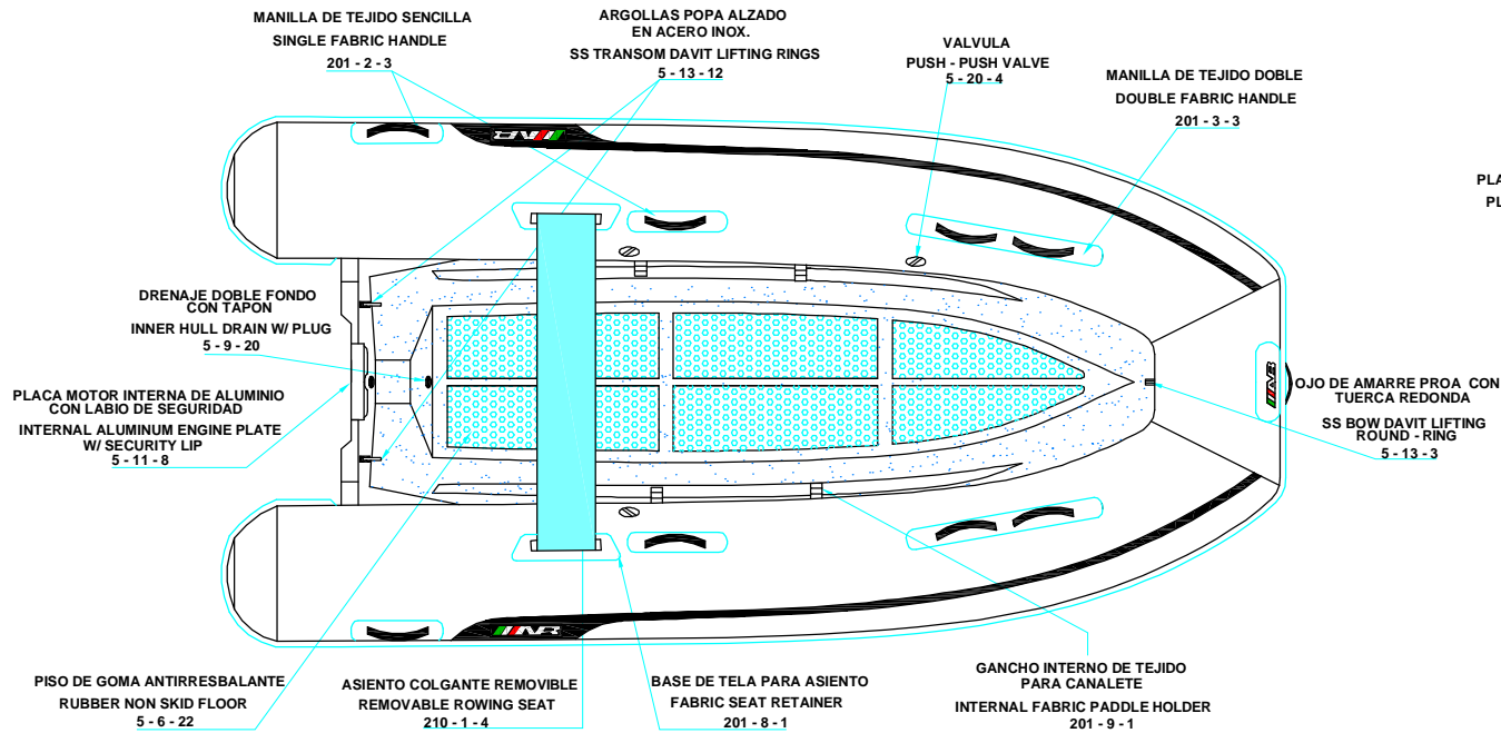
PLANT VIEW VISTA EN PLANTA
